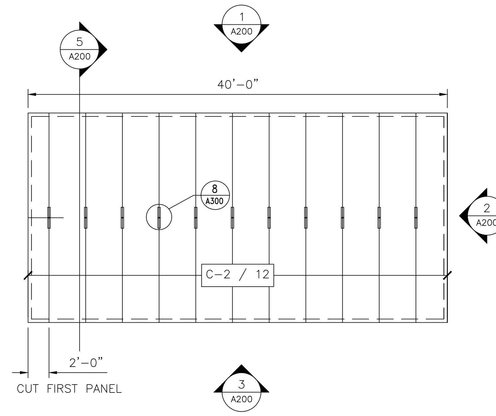
2 CEILING PLAN SCALE: N.T.S.
