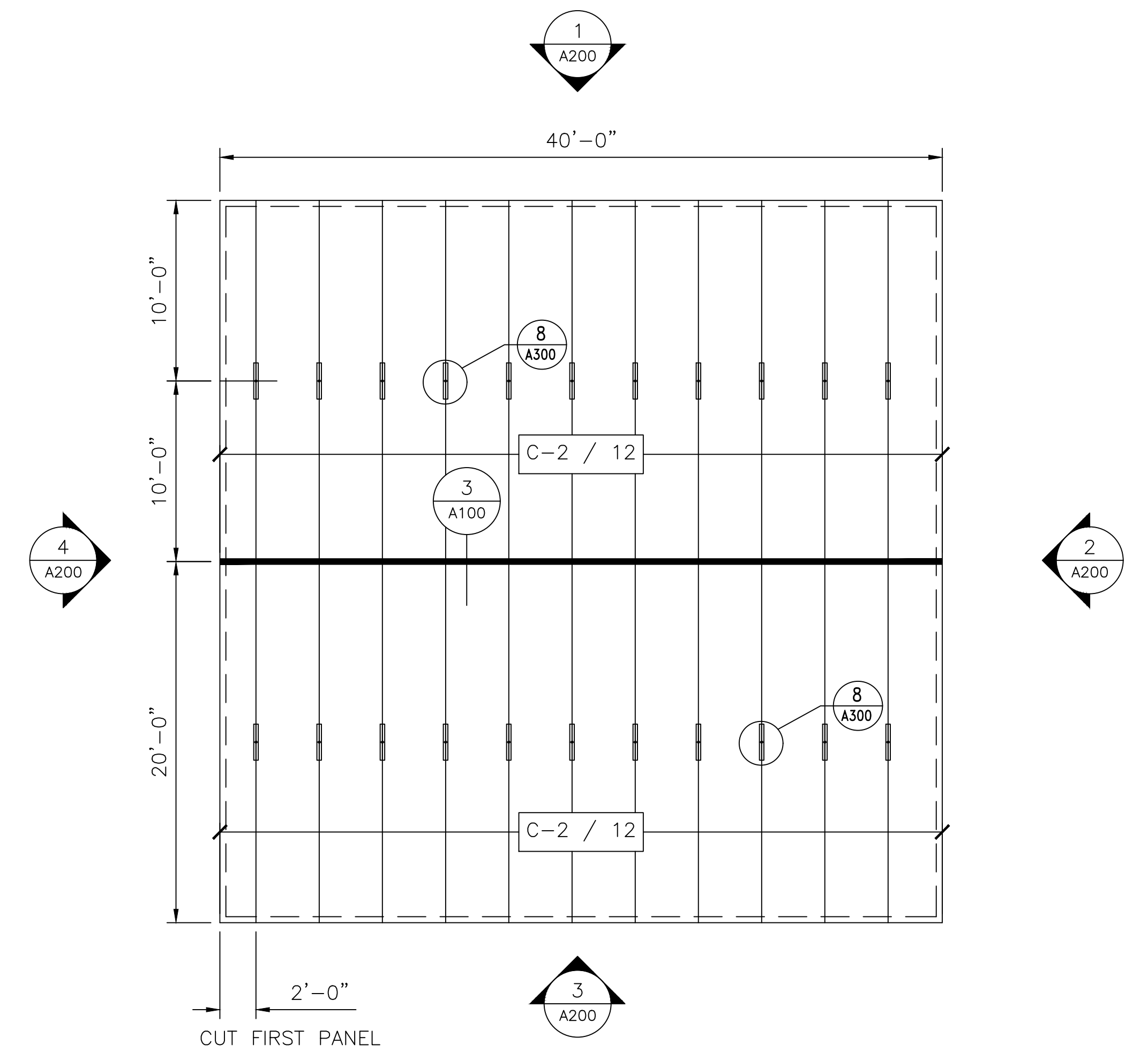
2 CEILING PLAN A100 SCALE: N.T.S.
